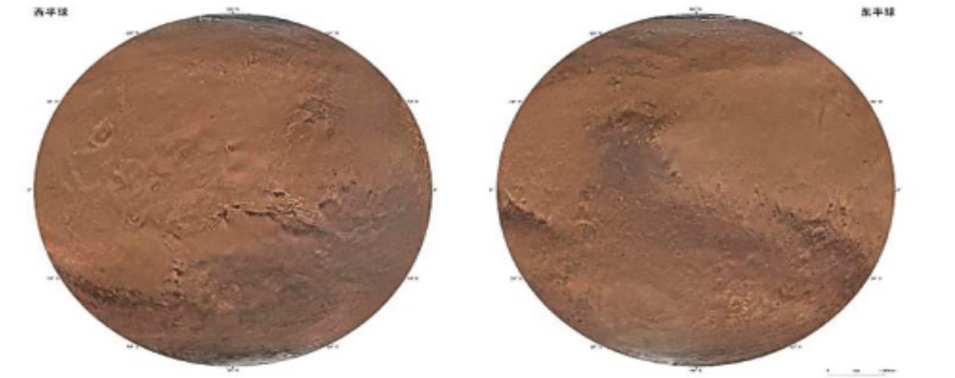
↑东西半球正射投影图(国家航天局提供)
